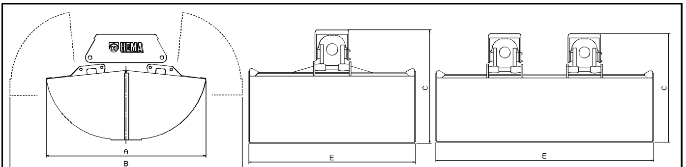
Korngrab KG 90-2000-2
