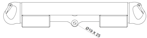
Center ophæng under åget \varnothing 19 \times 25 mm f. 3,25 T Sjækel
